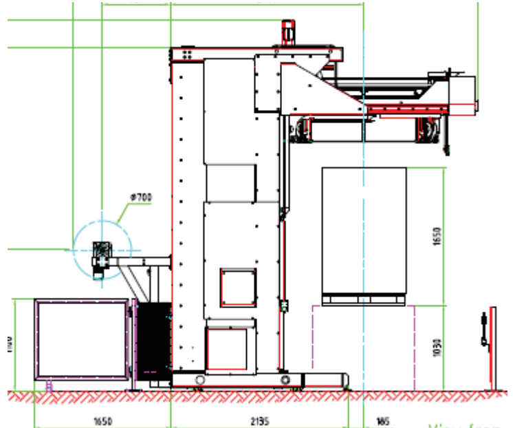
Haubenstretcher IS43
