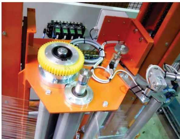
automatischer Dreharmwickler für Großpakete
