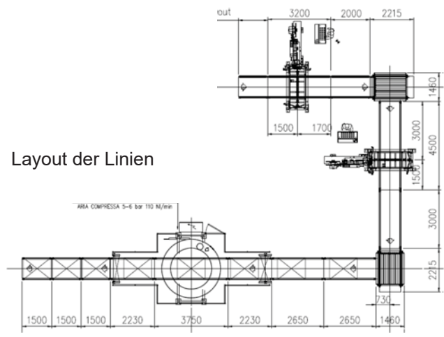
Seitenverschlussumreifung vor Wickler
