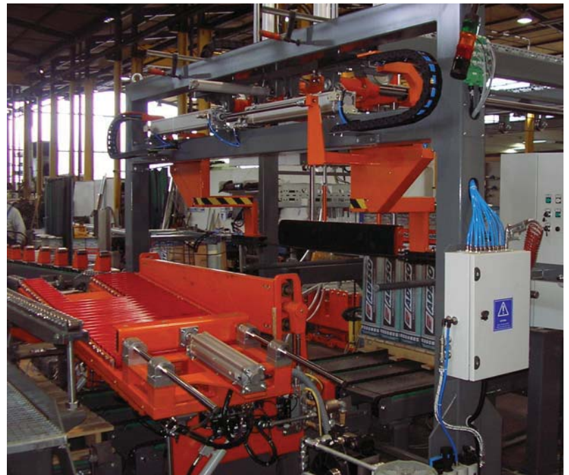
Einbausituation im Palettierer
