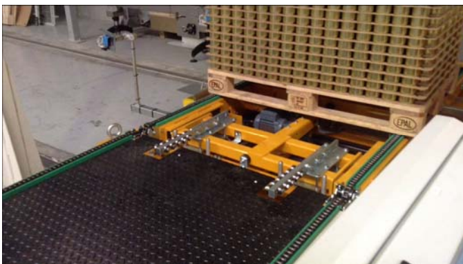
Ausfahrbare Übergangsrollen / Übergabe auf Shuttle 2
