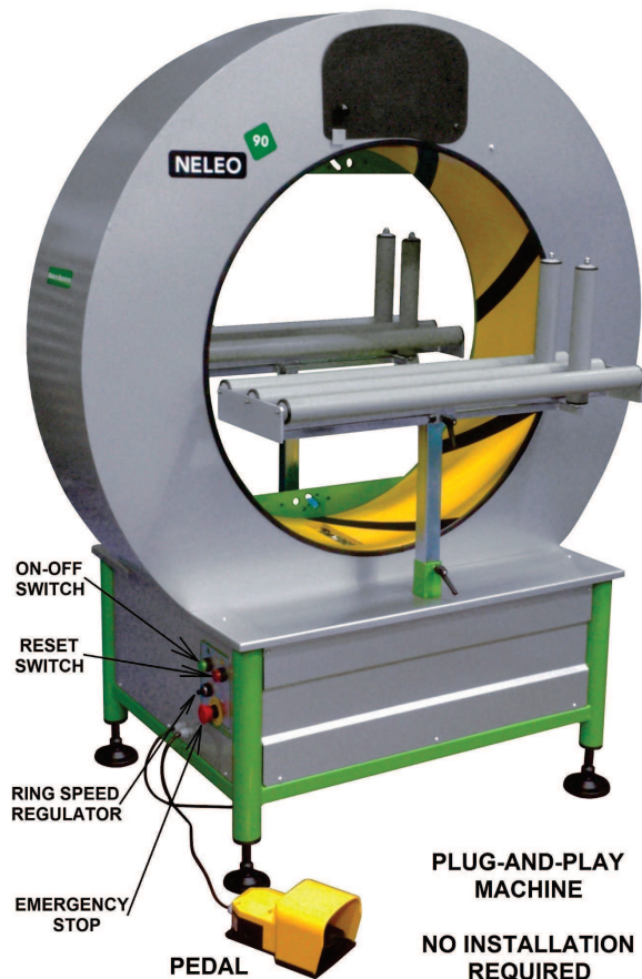
Horizontalwickelmaschine Neleo 90
