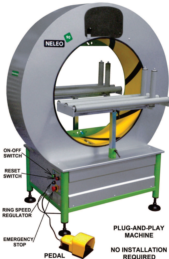
Horizontalwackelmaschine Neleo 90
