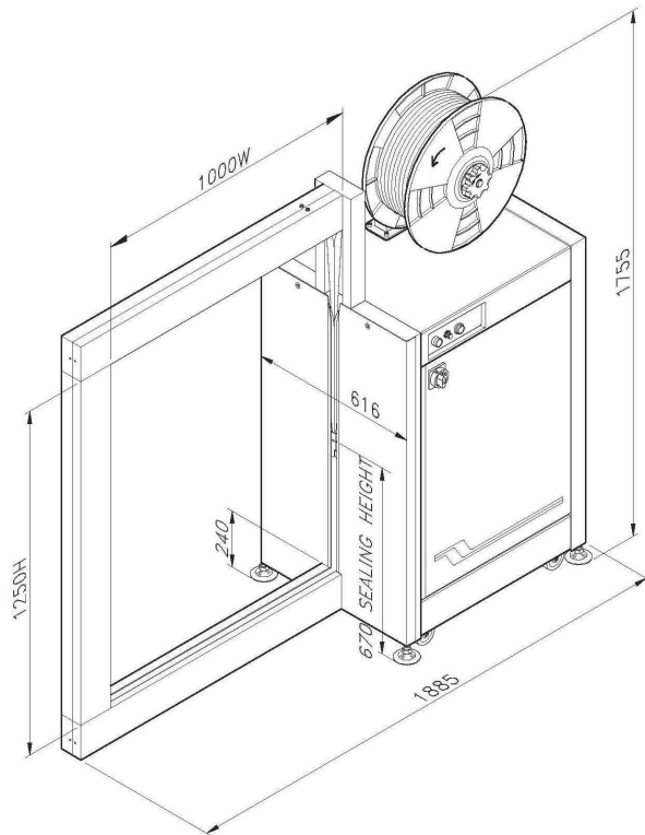
Automatische Umreifungsmaschine R62
