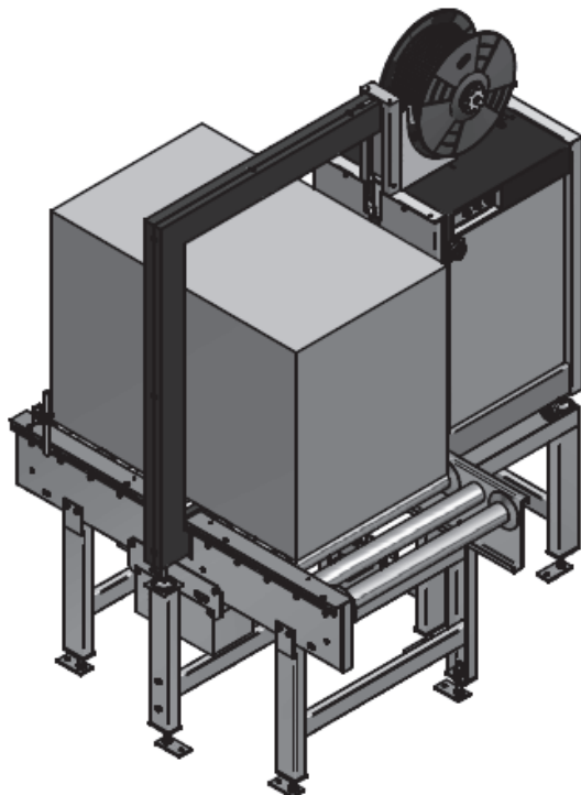
Automatische Umreifungsmaschine R62
