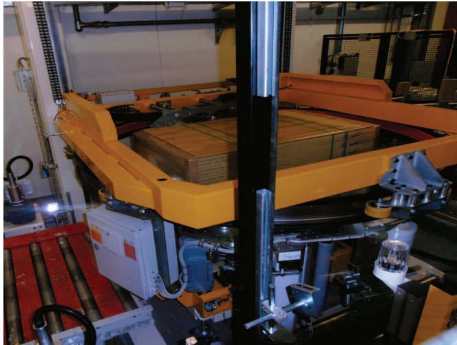
Umwicklungsvorgang
