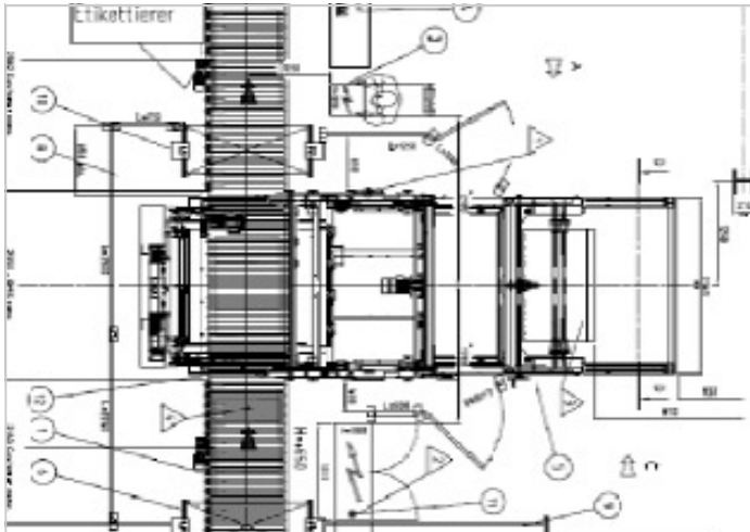
Layout der Maschine
