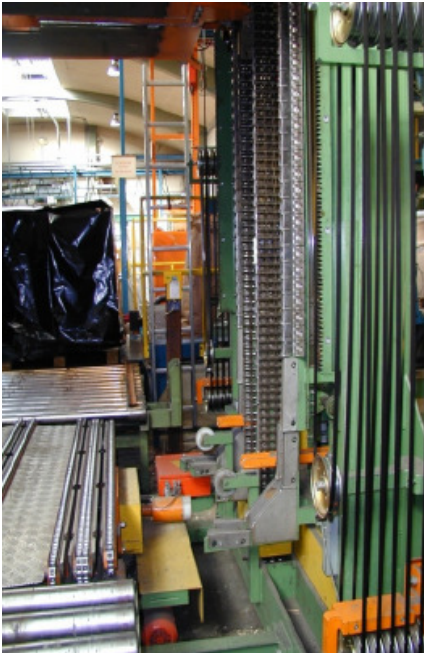
Vertikale Bandführungen mit Stahlbandabroller
