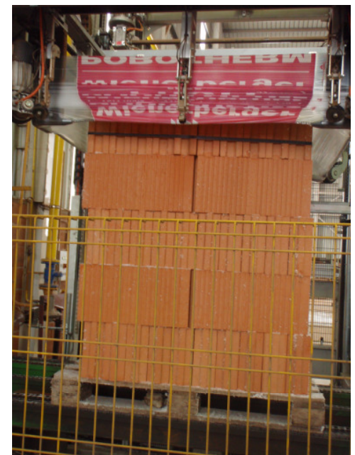
Abrollvorgang Haubenstretcher
