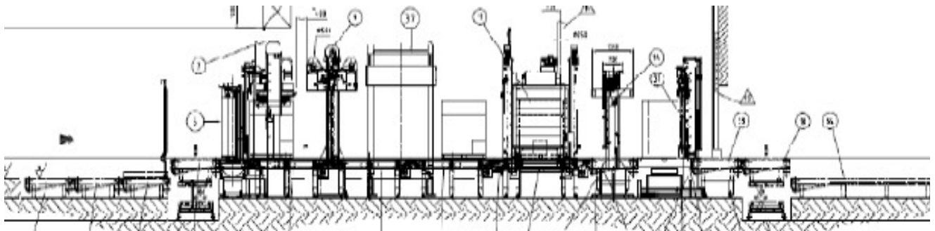
Linienaufbau: Vorhangsystem, Einschlagmaschine., Deckblatta., Haubenüberzieher, Ofen, Presse, Umreifung
