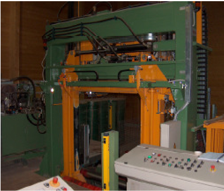
Maschine 2004: ausgestattet mit 4-fach Presse und Winkelanelger
